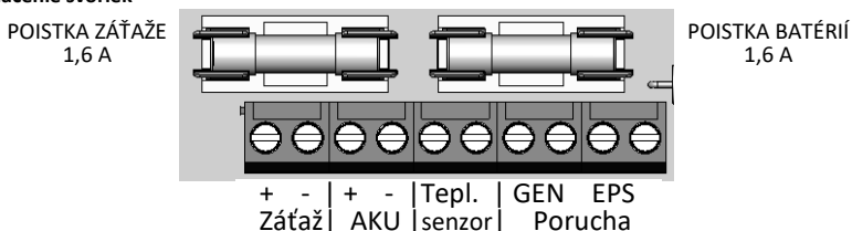
Obrázok 4 – Označenie svoriek
