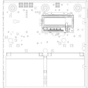
STV2402 in E-Box mit 17-Ah-Batterien
