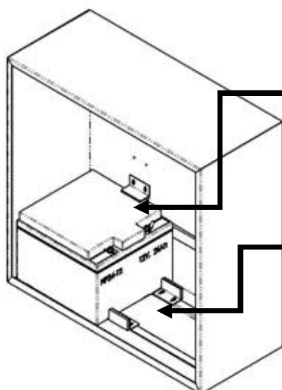
2402ST se skříní H a bateriemi 24Ah (baterie pro názornost vynechány)
