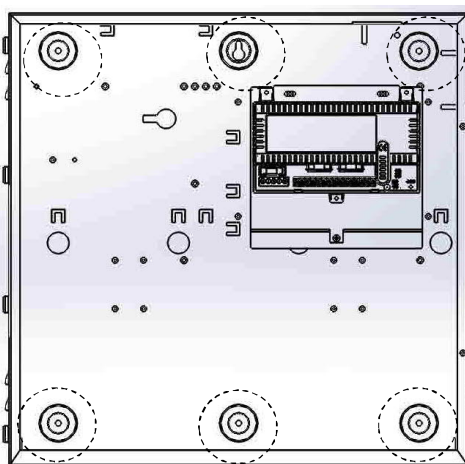
Kryt typu H
