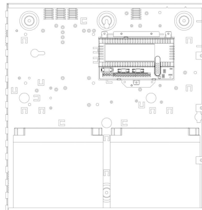
2402ST se skříní H a bateriemi 38Ah
