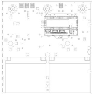
STV2405 dans un boîtier E avec batteries 17 Ah
