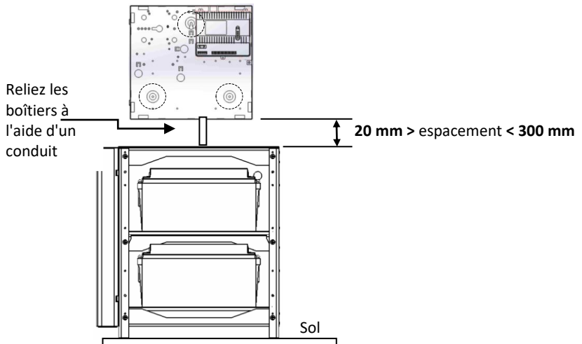
Figure 3 Utilisation du boîtier BATT-BOX-65
